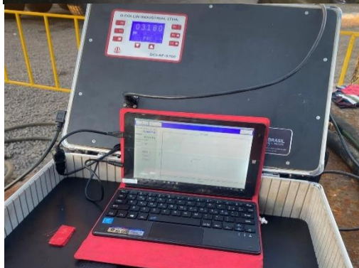
Teste Hidrostático
